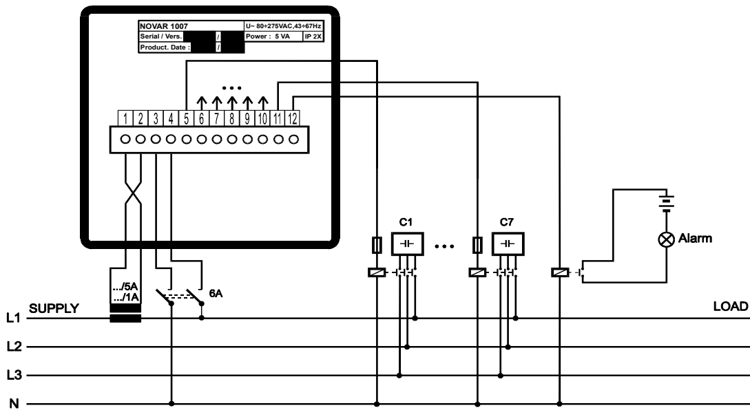
Novar 1007 – schemat podłączenia
