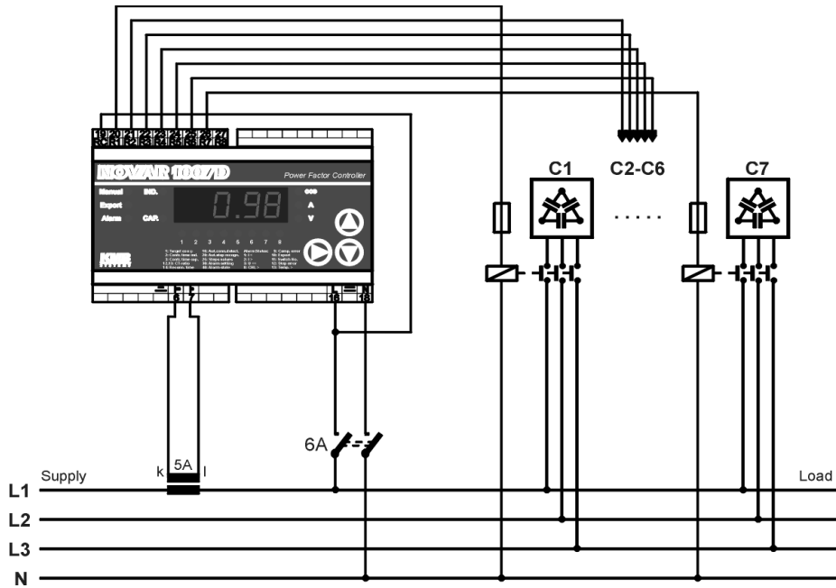
Novar 1007 – schemat podłączenia
